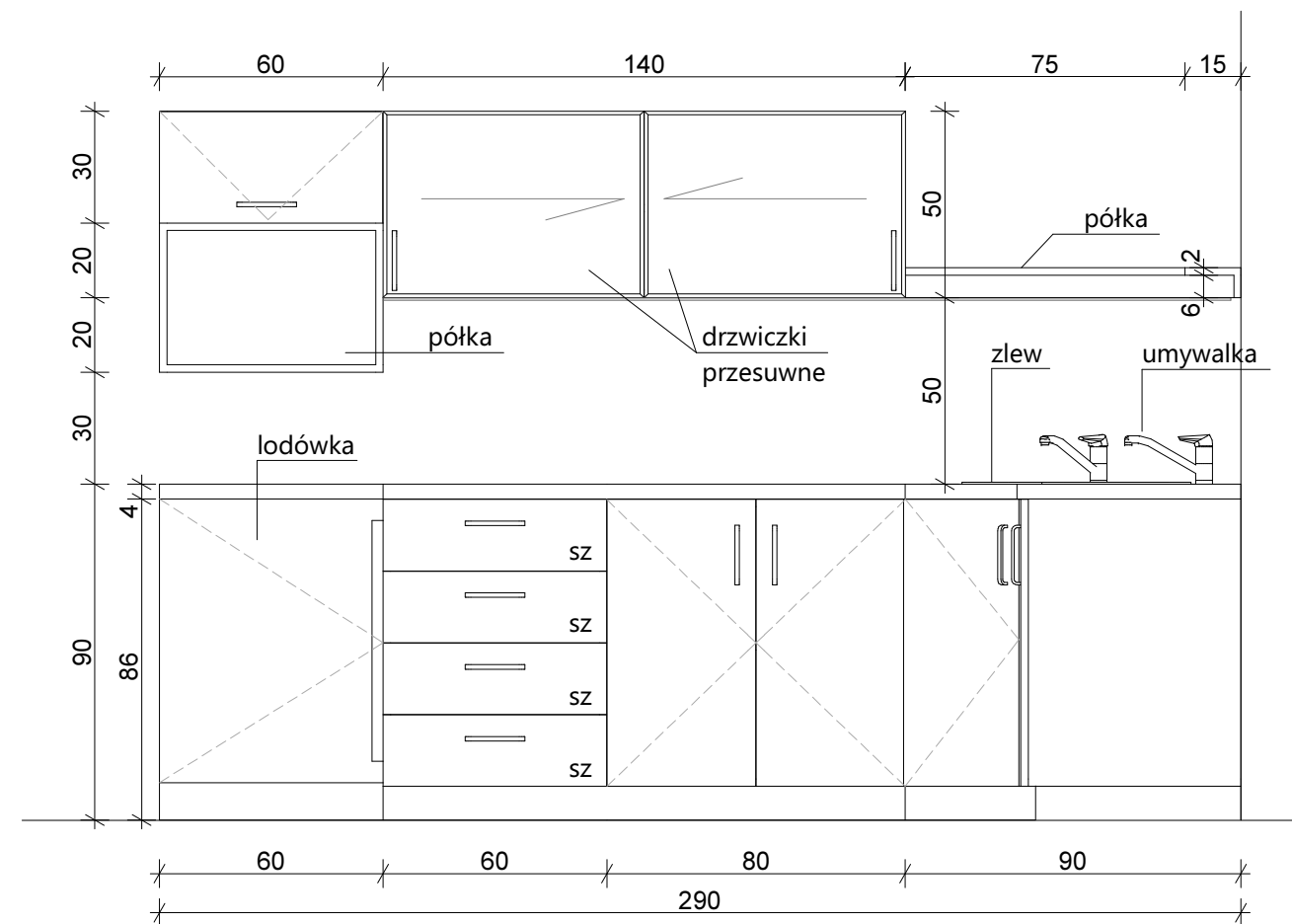
W1 przód 1:20
