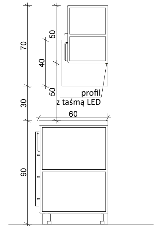
W4 przekrój 1:20
