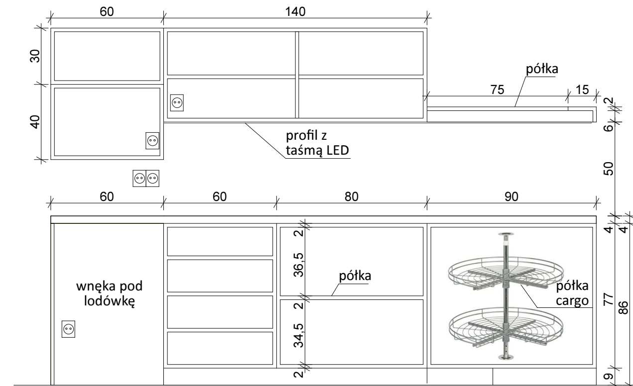
W3 przekrój 1:20
