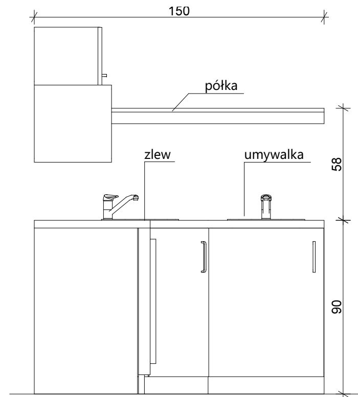
W2 z boku 1:20
